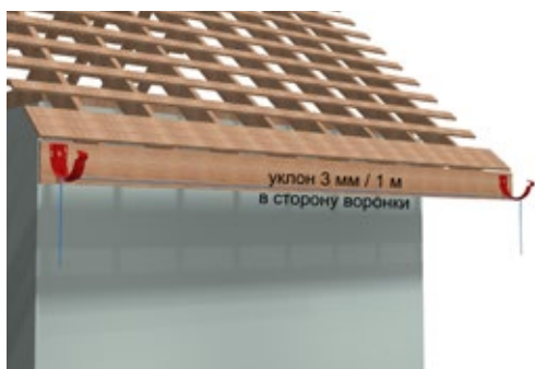
Рис. 7 Обеспечение уклона между крайними кронштейнами в сторону воронки
