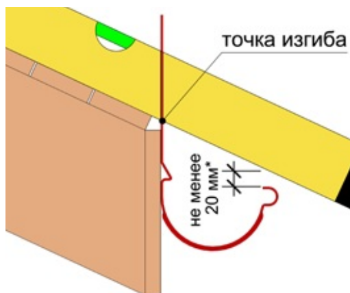
Рис. 3 Нахождение точки изгиба на самом верхнем кронштейне
